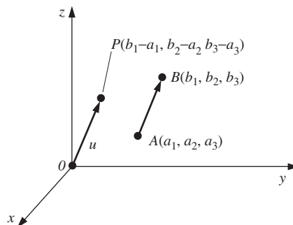
u = B - A
